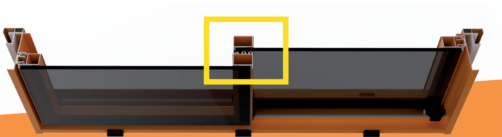
CORTE HORIZONTAL LADO EXTERNO
