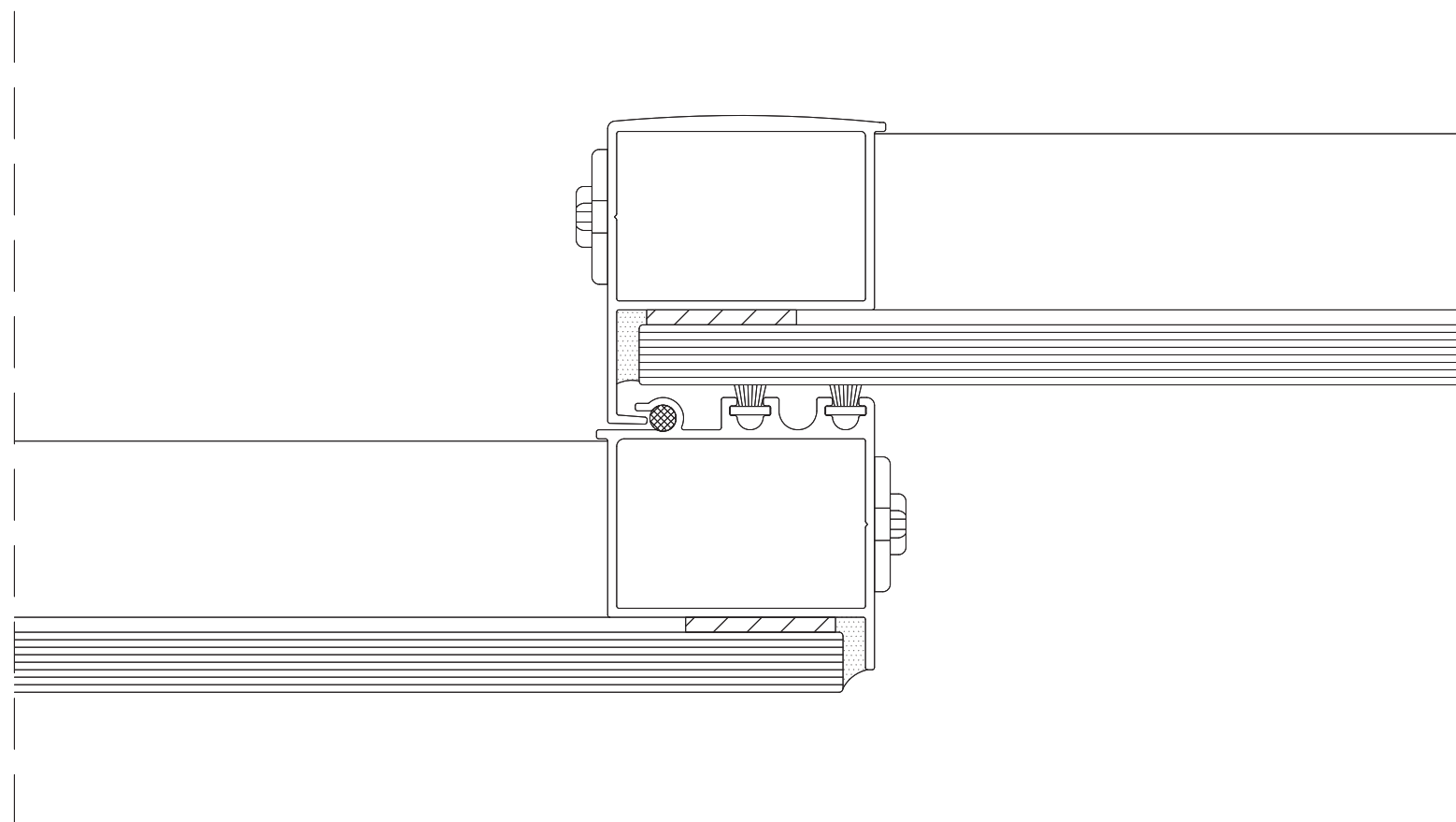
CORTE HORIZONTAL LADO EXTERNO
