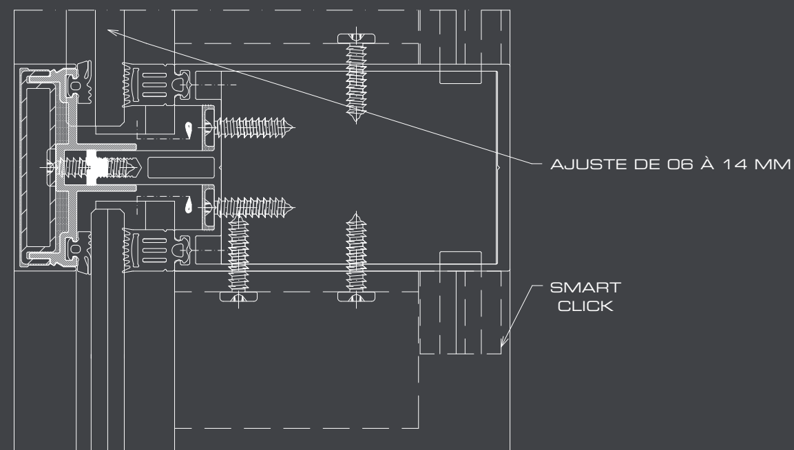
CORTE HORIZONTAL
