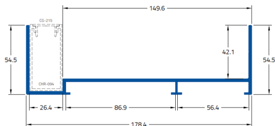
CM-807 Contramarco para Calha
