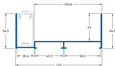
CM-806 Contramarco para Calha
